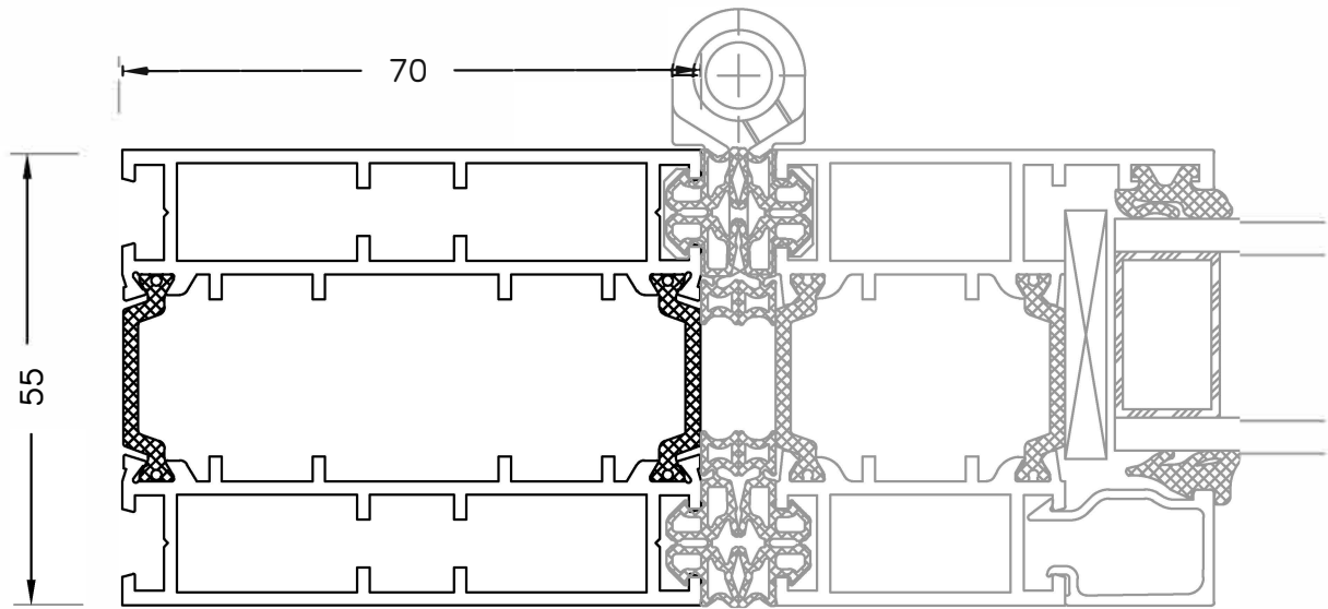
70mm Jamb
